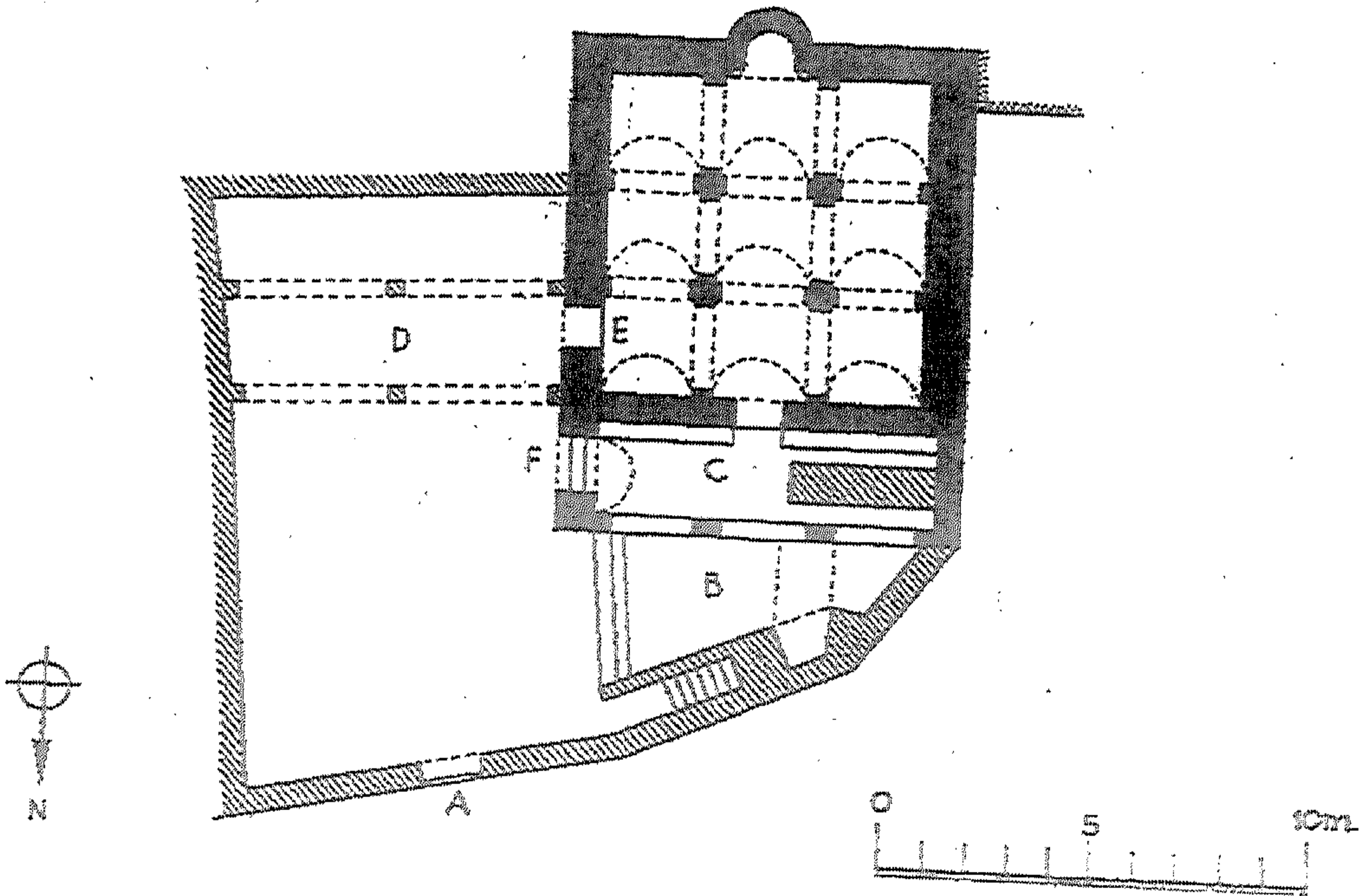
(شكل رقم ٣٤) رسم تخطيطى لجامع بوفتافة عن كرزويل.
